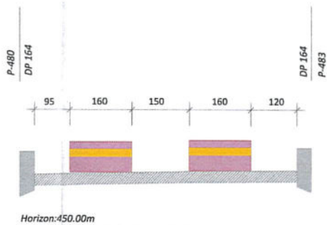
Coupe A-A'
